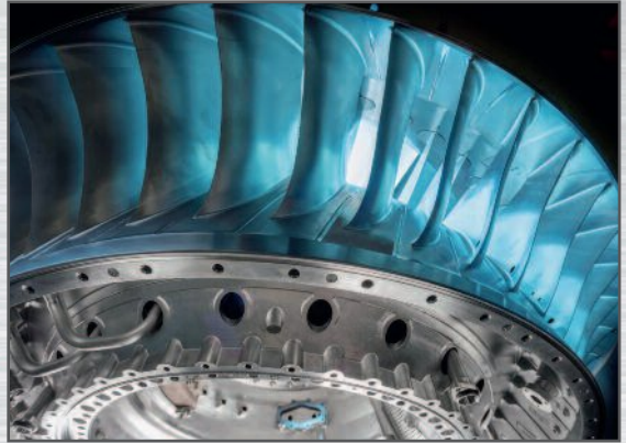
Additiv gefertigtes Lagergehäuse (Durchmesser 1,5 m) mit generativ gefertigten Schaufeln.
