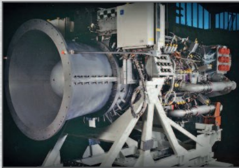
1993 – BR700-Kerntriebwerk.
