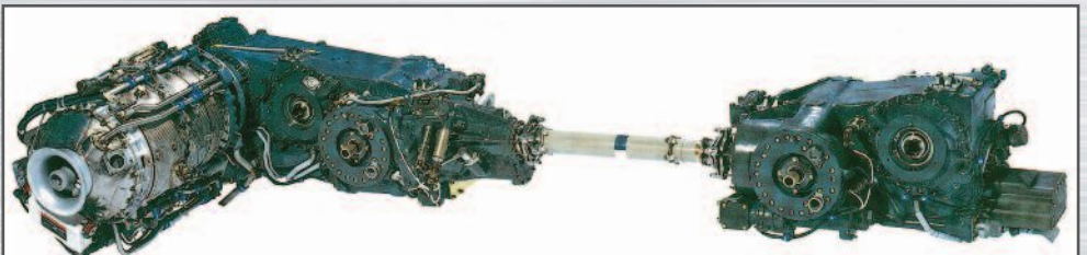
Secondary Power System für TORNADO.
